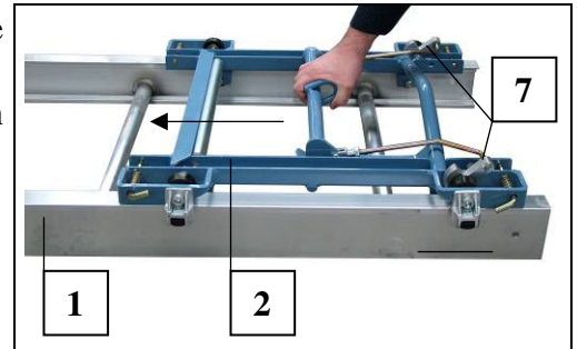
Fig. 18 Slede in het voetstuk schuiven
